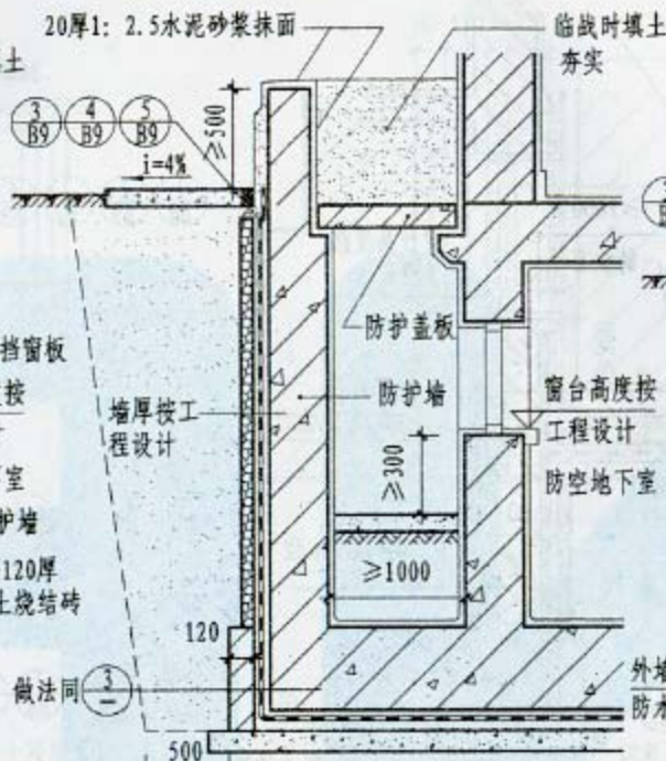
② 战时半填土窗井
