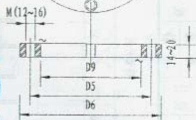
9 翼盘
