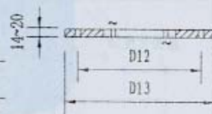
11 压环法兰
