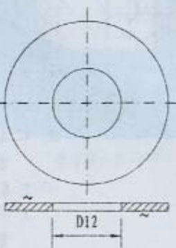
13 固定法兰盘
