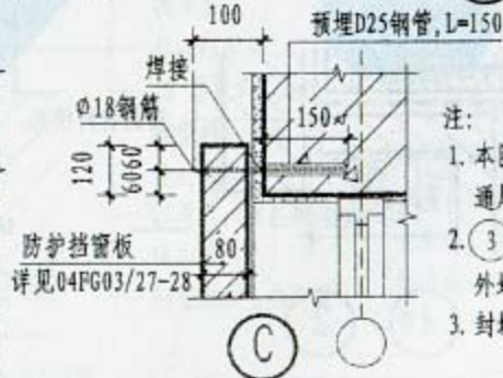
② 战时半填土窗井
