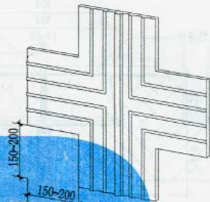
A 外贴式止水带在施工缝与变形缝相交处的专用配件
