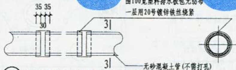
③ 平接式(无砂混凝土管)渗水管
