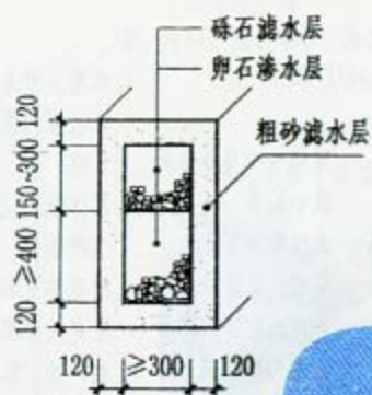
① 无管型
