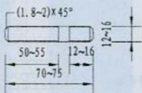
8 双头螺杆
