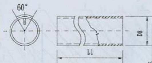
1 套管
