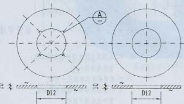
12 压毡环
