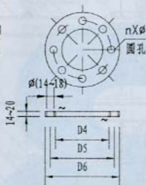
7 法兰盘
