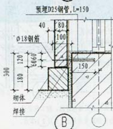
② 战时半填土窗井
