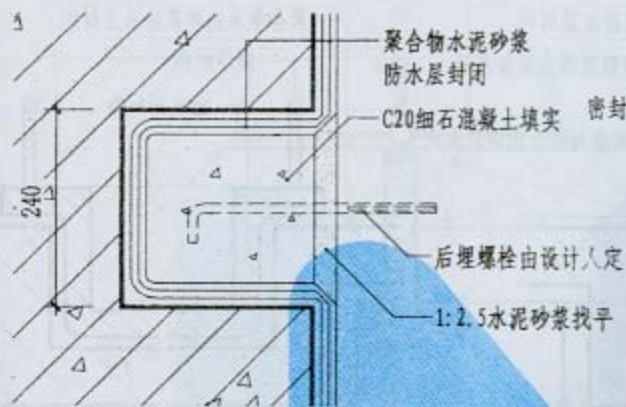
① 留洞后镶螺栓
