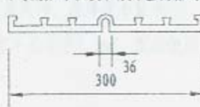
⑬ 橡胶或塑料止水带
