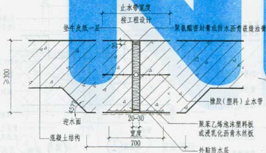
② 中埋式止水带与外贴防水层(止水带、防水卷材、防水涂料)复合使用
