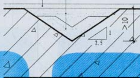
② 基层表面不平的处理
