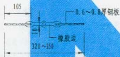
⑤ 钢边橡胶止水带
