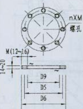
6 翼盘
